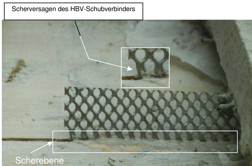
Abbildung 6: Scherversagen des HBV-Schubverbinders
