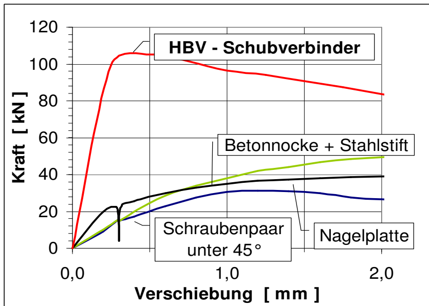
Abbildung 7: Kraft-Verschiebungs-Diagramm unterschiedlicher Verbindungsmittel
