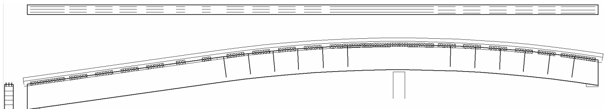
Abbildung 9: Anordnung der HBV-Schubverbinder und konstruktive Quersicherung
